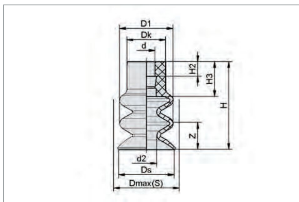
TGB-12至25
